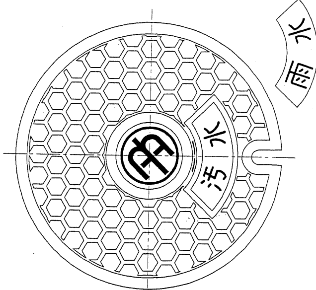
1 カバー平面図
