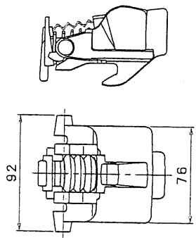
5 自動錠詳細図
